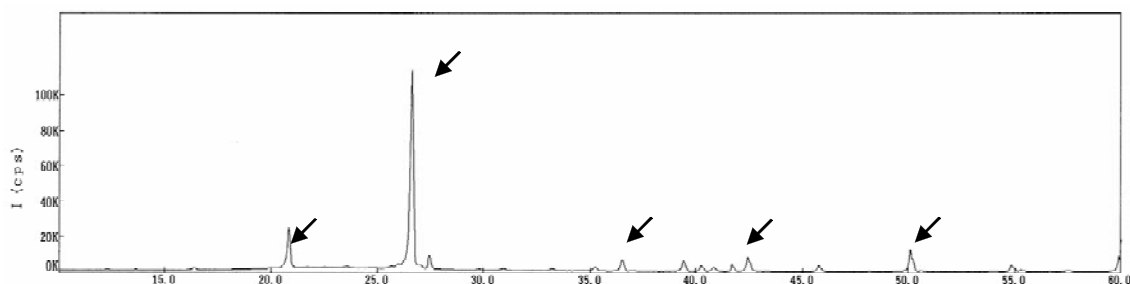
図 2 X線回折 (←はSiO 2 の主なピークを示す。)
